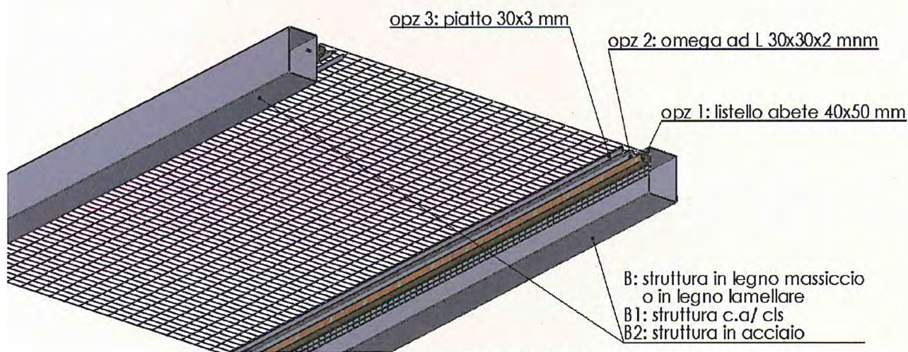
Fig. 9: Schema di posa B, B1, B2
