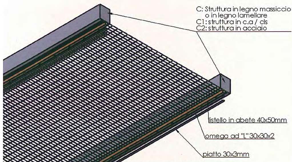
Fig. 10: schemi di posa C, C1, C2
